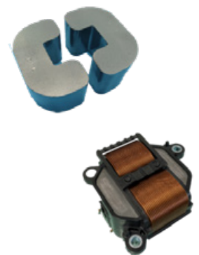
リアクトルコア
