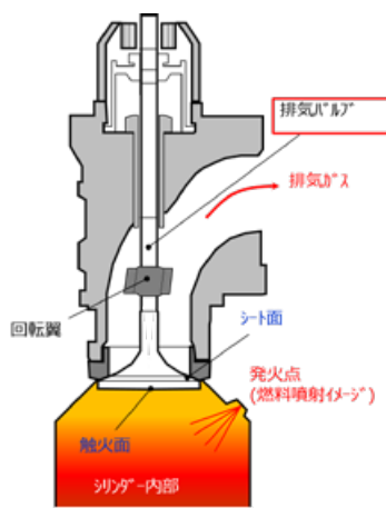
船舶機関の構造
