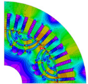
三層円弧磁石モータの解析例
