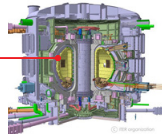
ITER 概念図
