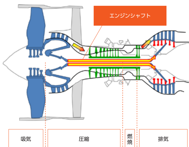
■ GEnx エンジン (イメージ図)
