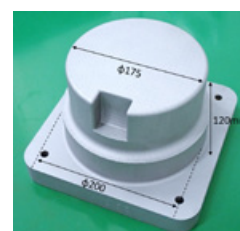
LTX™を用いた模擬型造形例
