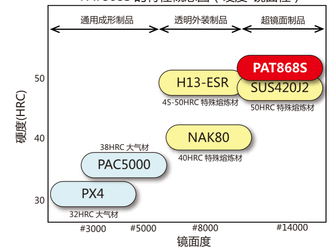
PAT868S 的特性概念图 (硬度-镜面性)
